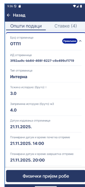
Слика 23: Приказ општих података улазне отпремнице
